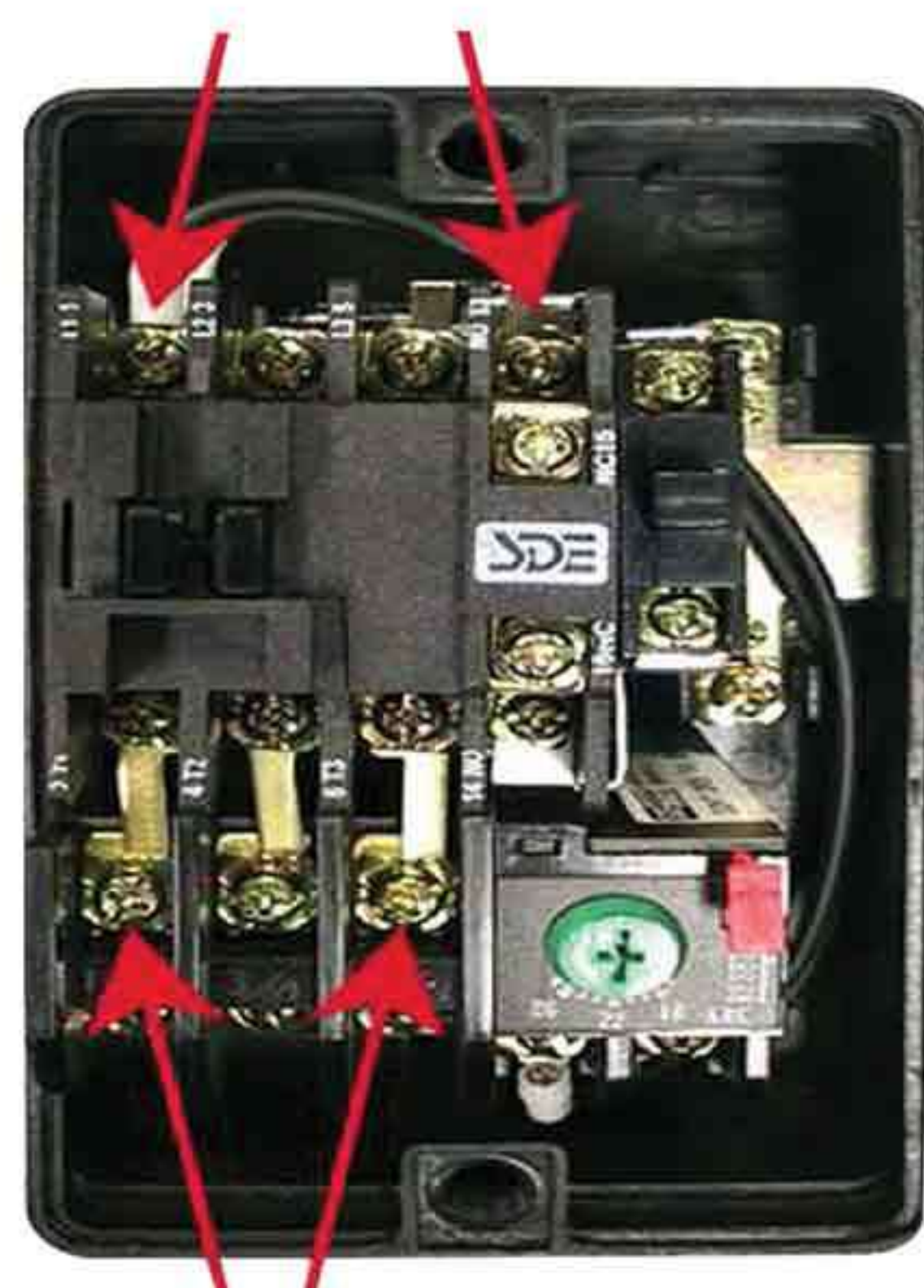
Motor Load
